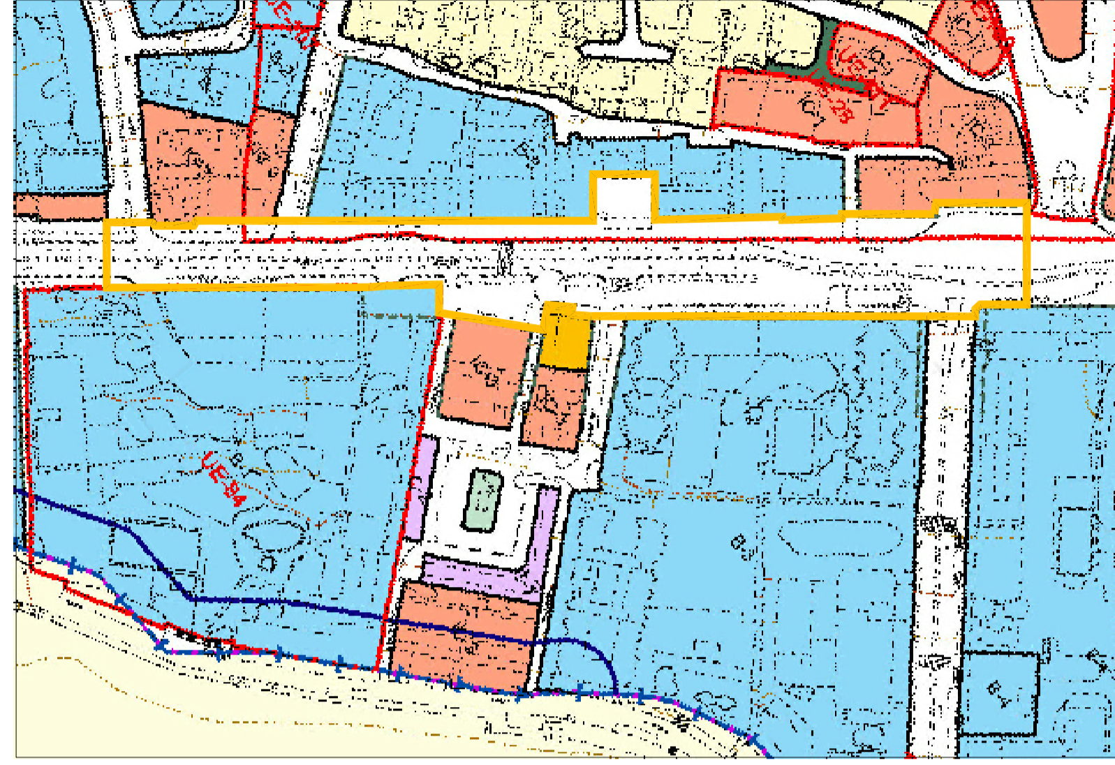
PLANO DE CALIFICACIÓN URBANA, ESCALA 1:2000
